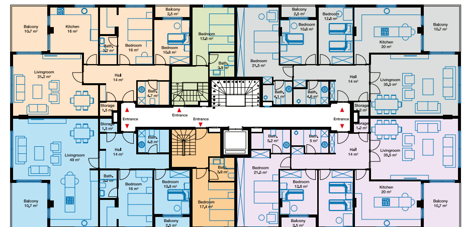
ПЛАН ПЕРВОГО ЭТАЖА ПЕНТХАУЗА
