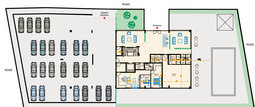
ПЛАН ЦОКОЛЬНОГО ЭТАЖА
